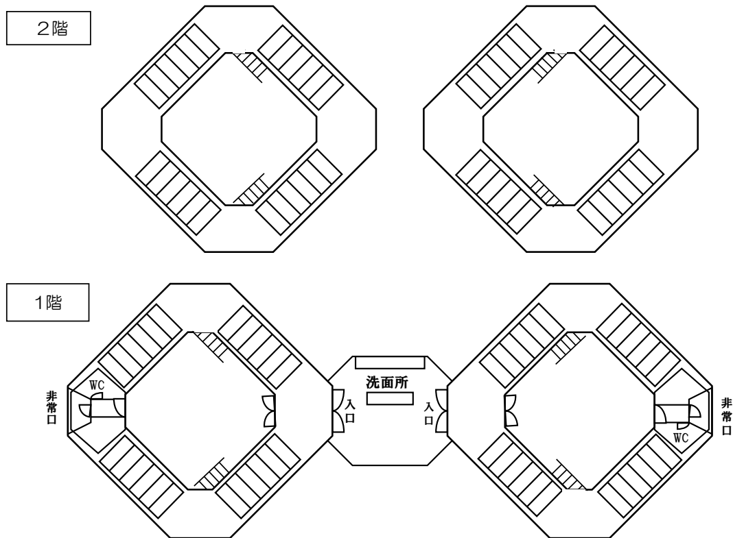
<青少年宿泊研修棟平面図>
